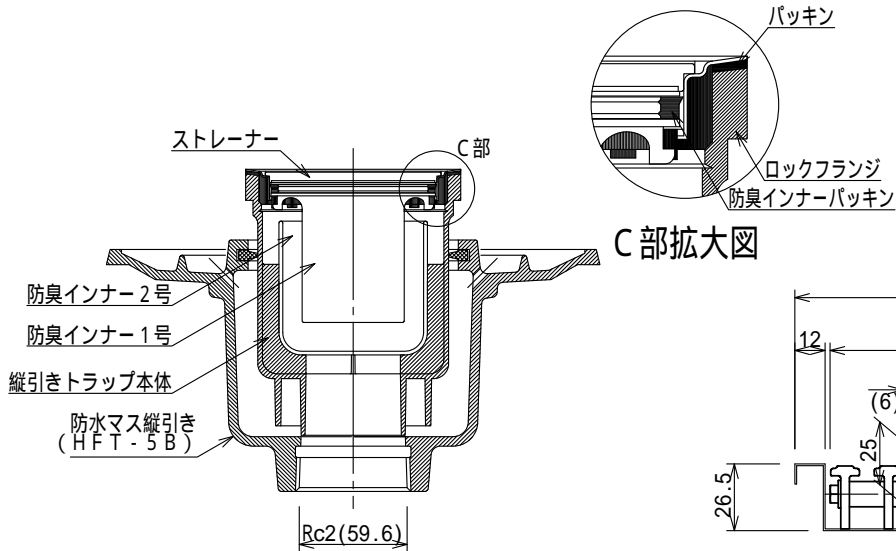
排水部詳細図 S=1:4
