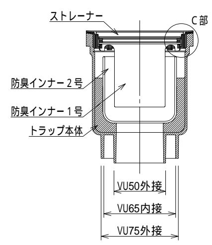
排水部詳細図 S=1:4
