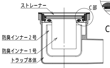
排水部詳細図 S=1:4
