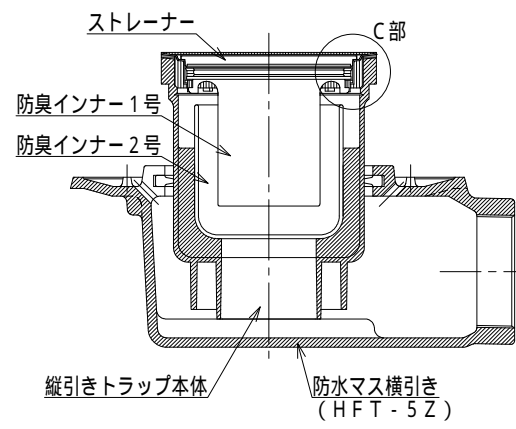
排水部詳細図 S=1:4
