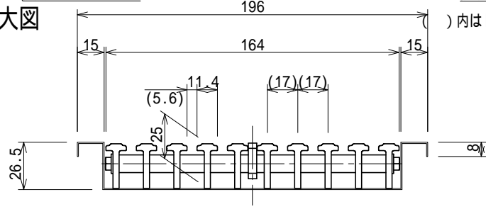
断面詳細図 S=1:3
