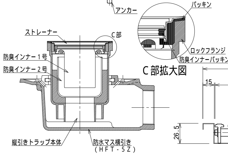
排水部詳細図 S=1:4
