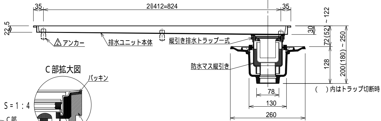
断面図
