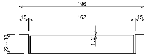
断面図
