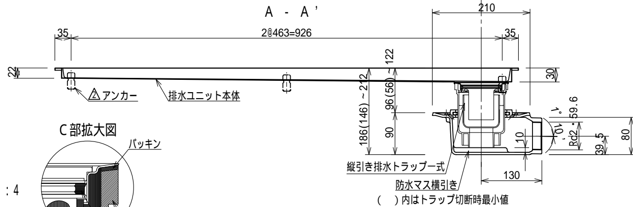
断面図
