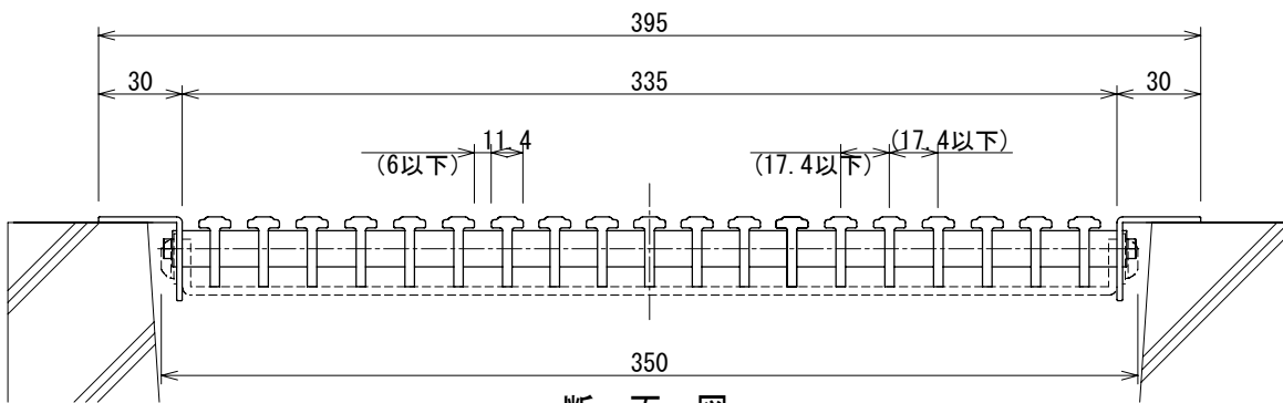
断面図 S=1:3
