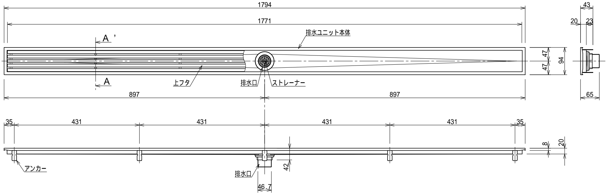
排水部詳細図 S=1:2
