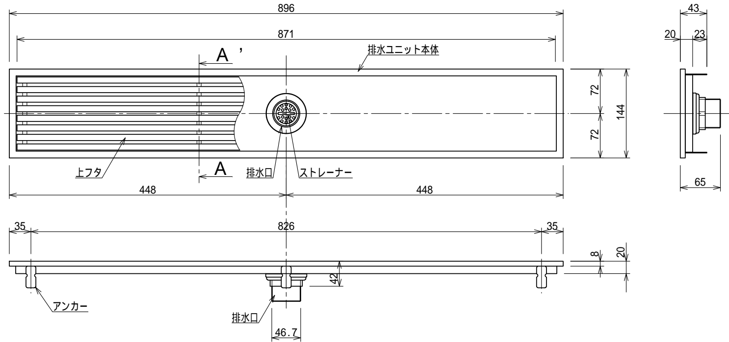
排水部詳細図 S=1:2
