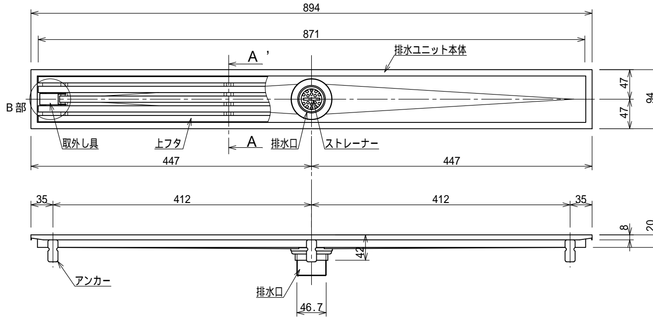
排水部詳細図 S=1:2
