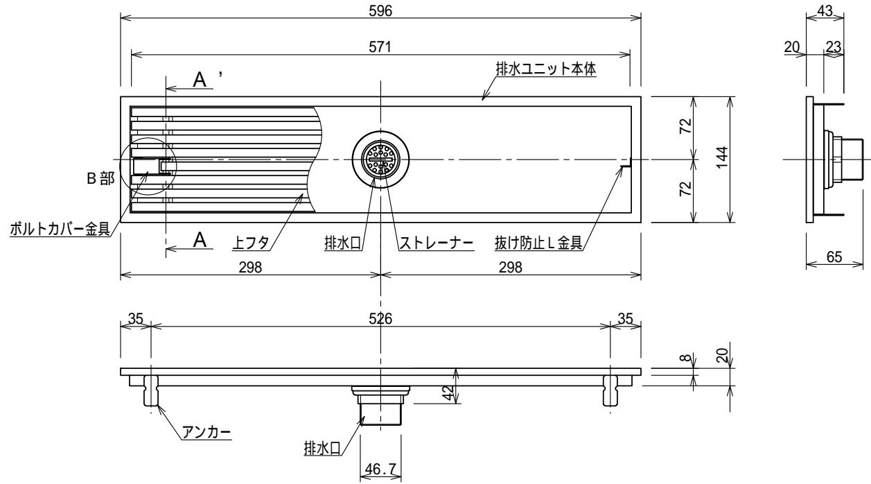
排水部詳細図 S=1:2
