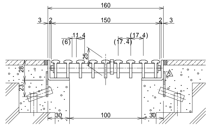
断面詳細図 S=1:3
