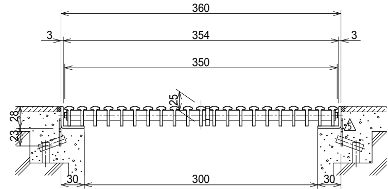
断面詳細図 S=1:5
