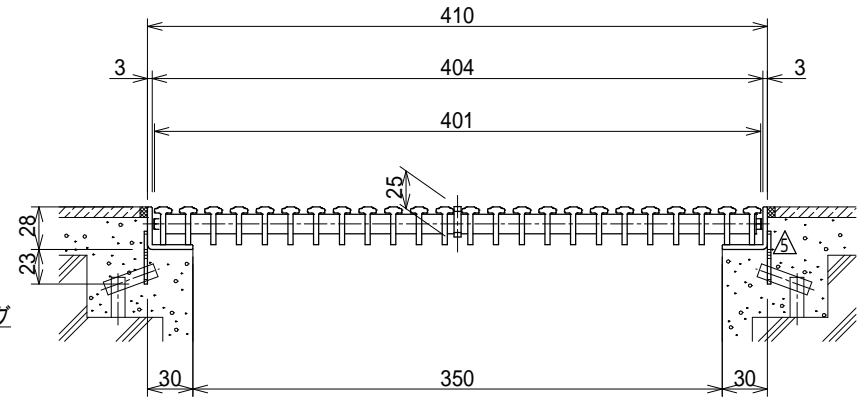
断面詳細図 S=1:5
