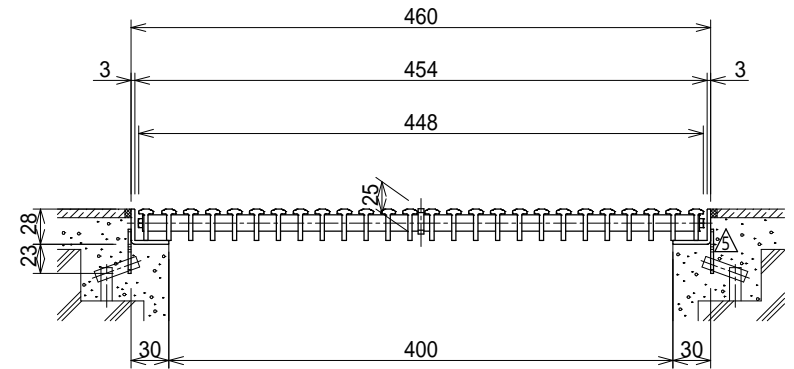
断面詳細図 S=1:6
