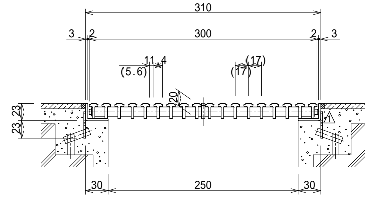
断面詳細図 S = 1 : 5
