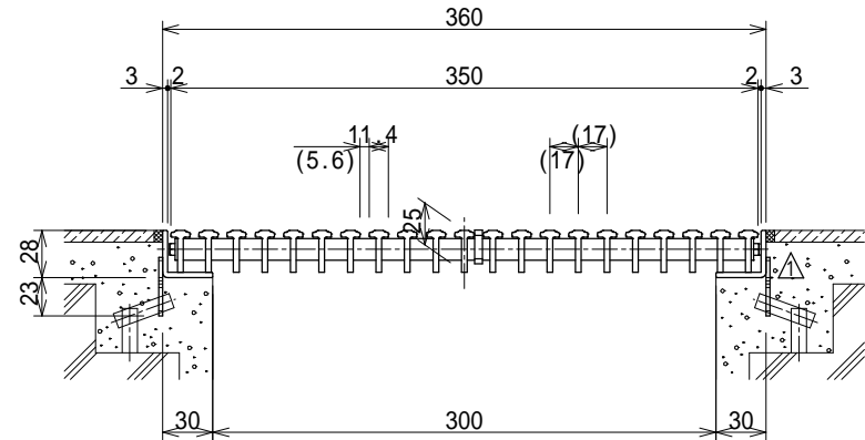
断面詳細図 S=1:5
