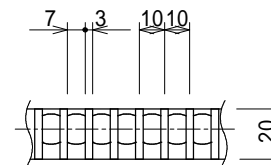
側面詳細図
