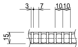
側面詳細 S = 1 : 3
