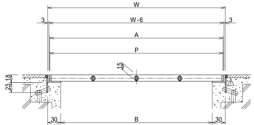
断面詳細図 S = 1 : 5
