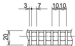
側面詳細 S=1:3
