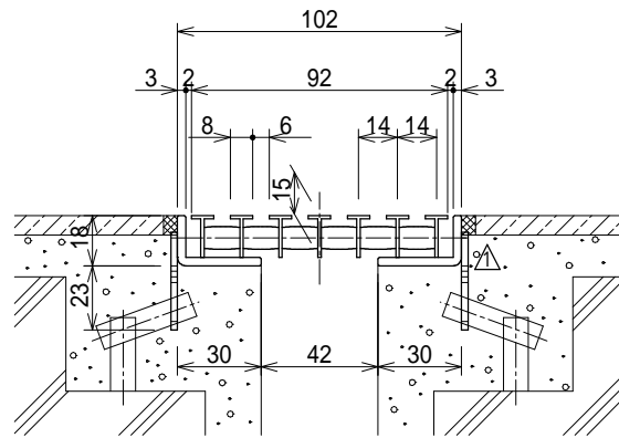
断面詳細図 S=1:3
