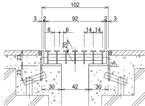
断面詳細図 S=1:3
