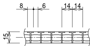
側面詳細 S = 1 : 3
