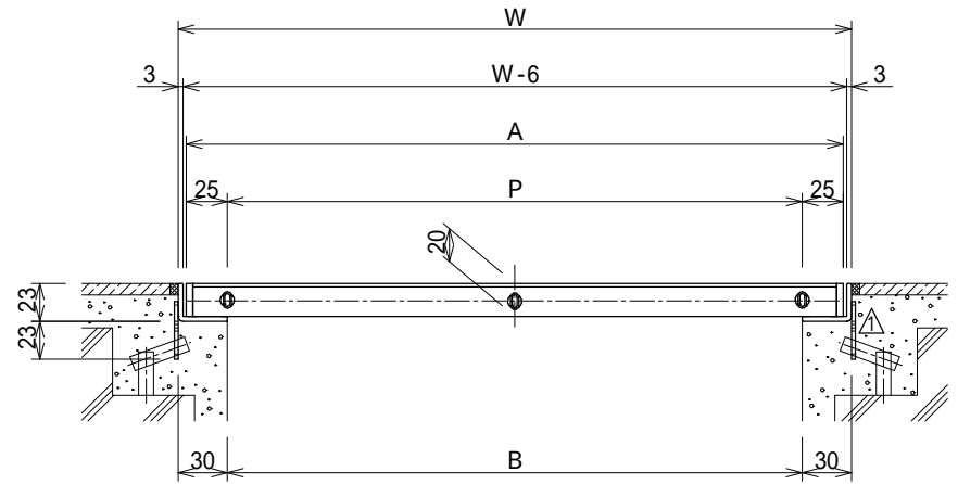
断面詳細図 S = 1 : 5
