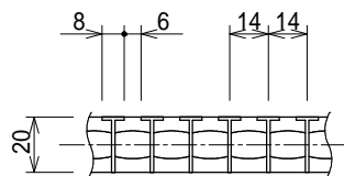
側面詳細 S = 1 : 3
