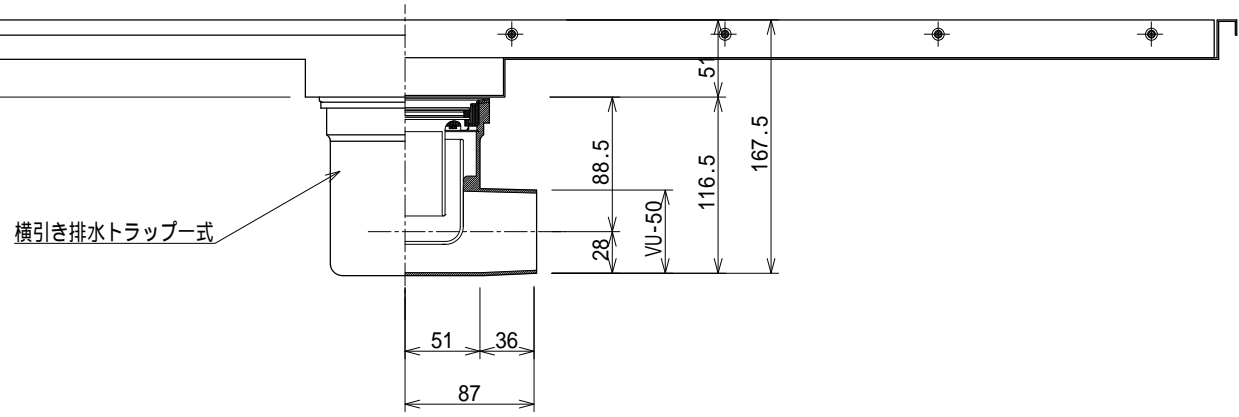
A - A' 断面図 S=1:3
